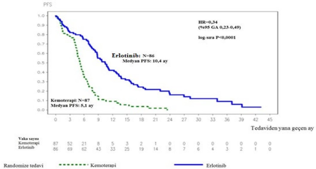
Şekil 1: ML20650 (EURTAC) çalışmasında araştırmacı tarafından değerlendirilen PFS için Kaplan-Meier eğrisi (Nisan 2012 kesimli)
